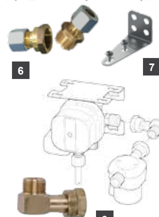
MonoControl CS, με γωνιακή βίδα 90° και φίλτρο υγραερίου
